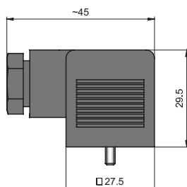
SCK-006 (Gerätestecker)
