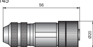
Einzelstecker SCK-145
