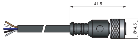
Anschlusskabel SCK-400-xx-45
