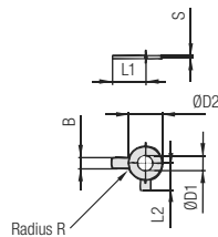
Sicherungsblech SI
