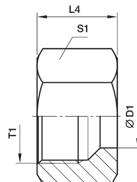
Überwurfmutter: M
