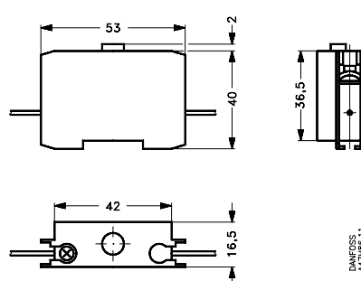
Elektronischer Timer ETB mit Clip
