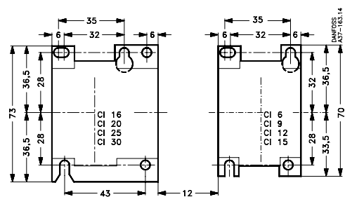
CI 6 – CI 30 mit mechanischer Verriegelung Bohrmaße
