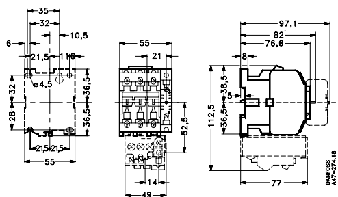
Schütze und Motorschalter CI 16, 20, 25, 30 Bohrmaße
