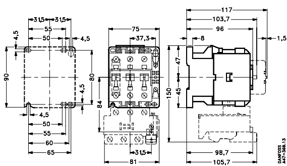
Schütze und Motorschalter CI 32, 37, 45, 50 Bohrmaße
