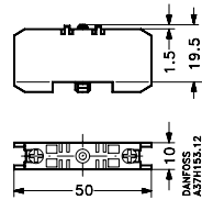
Elektronischer Timer ETB mit Clip
