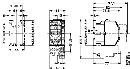
Schütze und Motorschalter CI 16, 20, 25, 30 Bohrmaße
