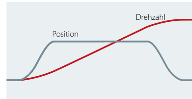
Abb. 2. Bewegungsprofil mit S-Rampen
