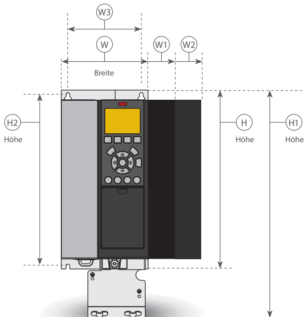
A3 IP 20 mit Option C
