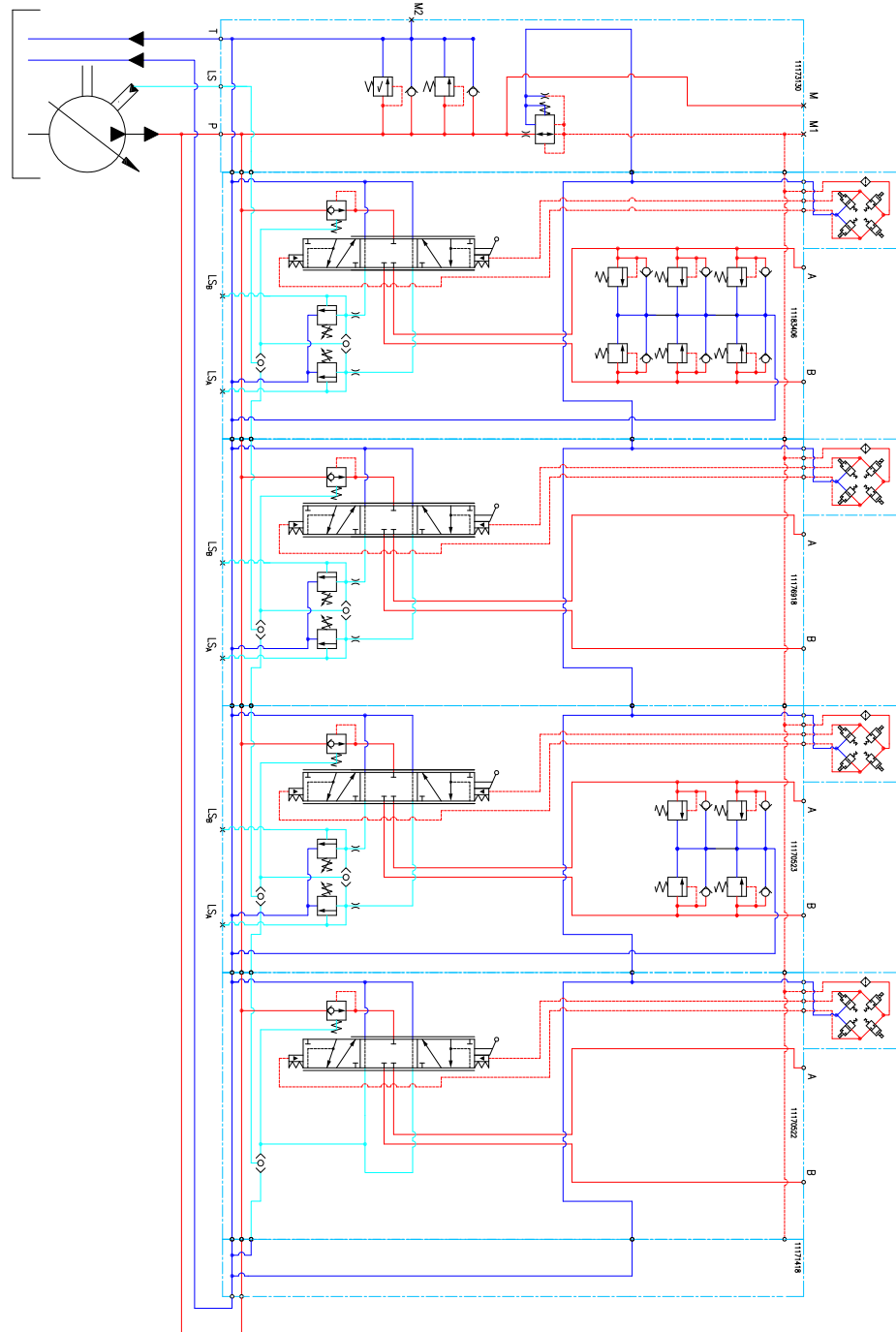
PVG 128/256 mit Endplatte mit P- und T-Anschluss
