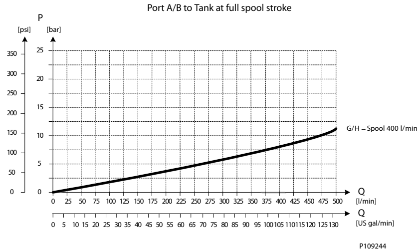
PVB 256 Kennlinie Rücklauf
