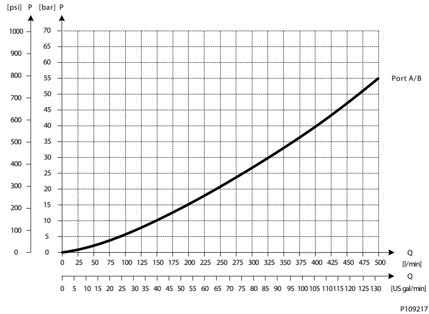
Lastunabhängiger Ölfluss, druckkompensiert
