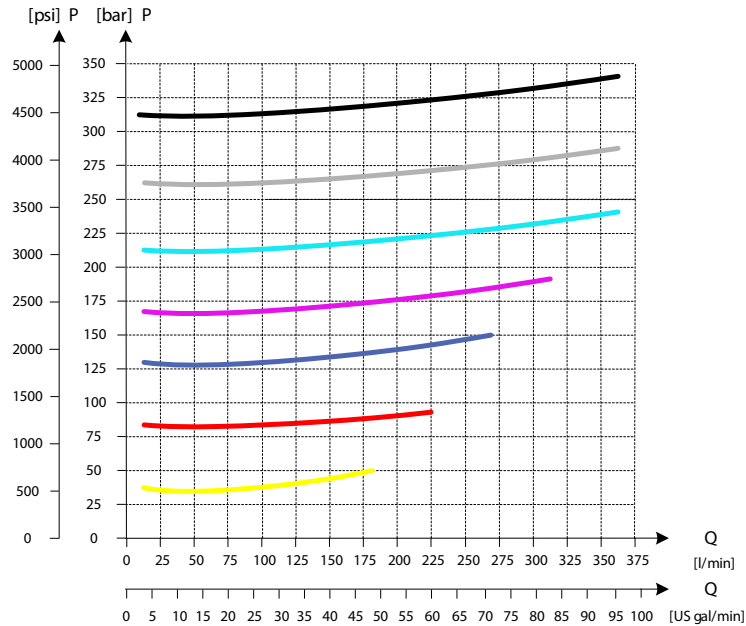
Drei PVLP-Schockventile
