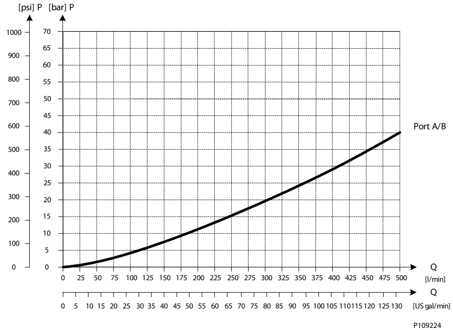
LS A/B -Druckbegrenzung
