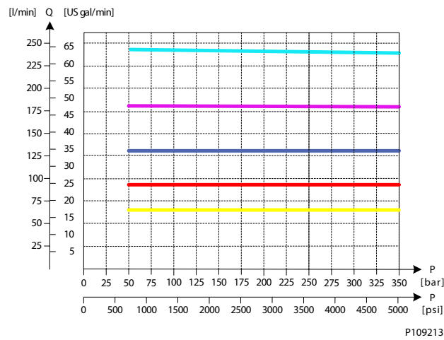
Lastunabhängiger Ölfluss, druckkompensiert
