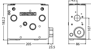
PVB 256 inlet module dimensions (mm)
