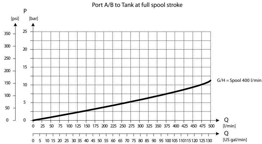
PVB 256 Kennlinie Rücklauf
