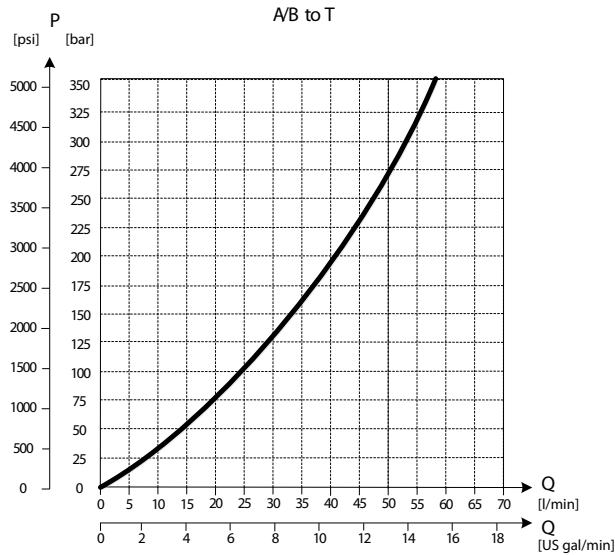
Druckabfall für offenen Schieber in Neutralstellung
