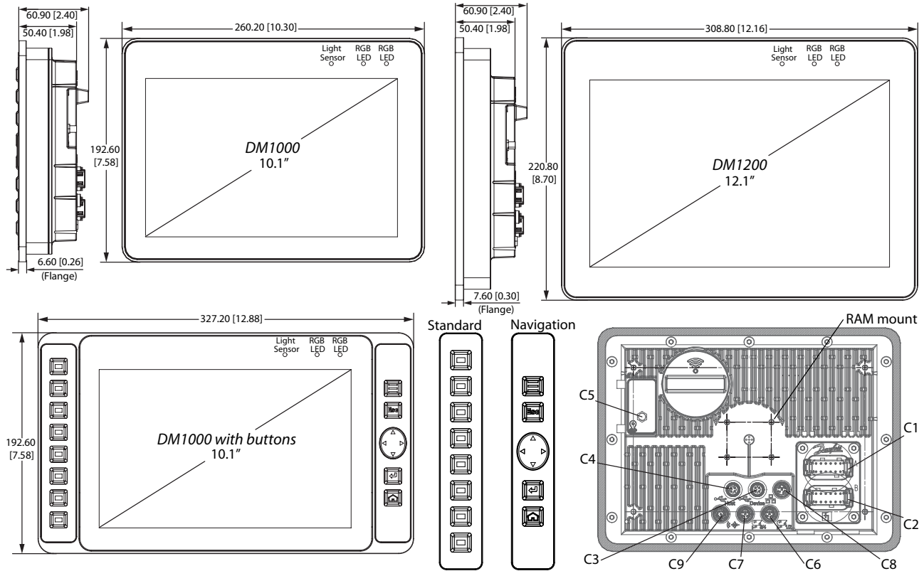
C1—DEUTSCH DTM06-12SA
