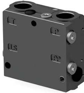
PVP Inlet Module
