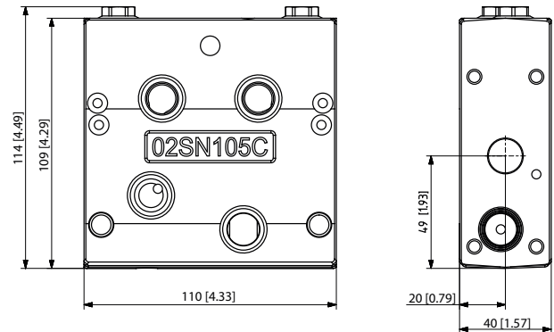
PVB 16 dimensions
