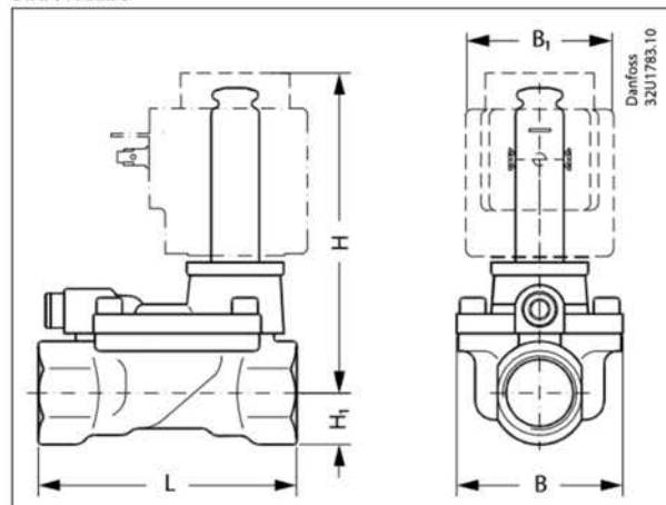
Bild 7: Maße
