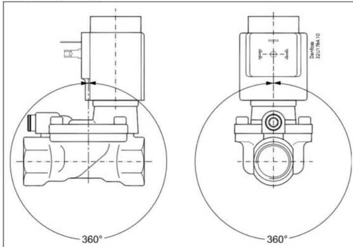
Bild 8: Montagewinkel
