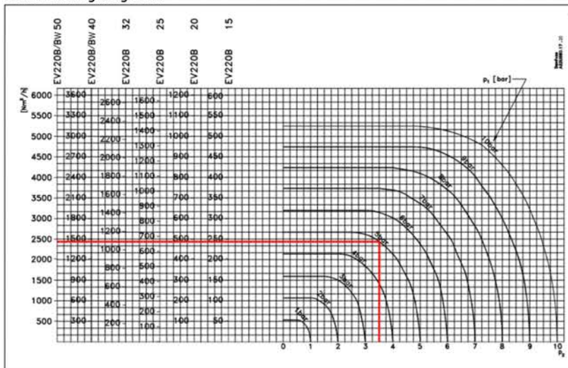
Bild 6: Leistungsdiagramm
