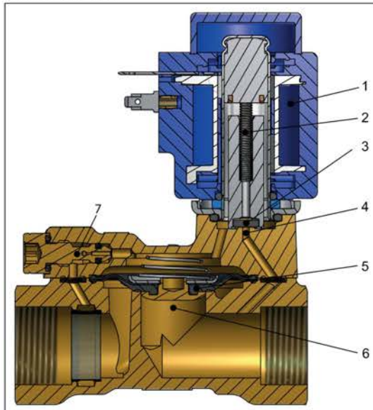
Bild 1: Funktion, NC
