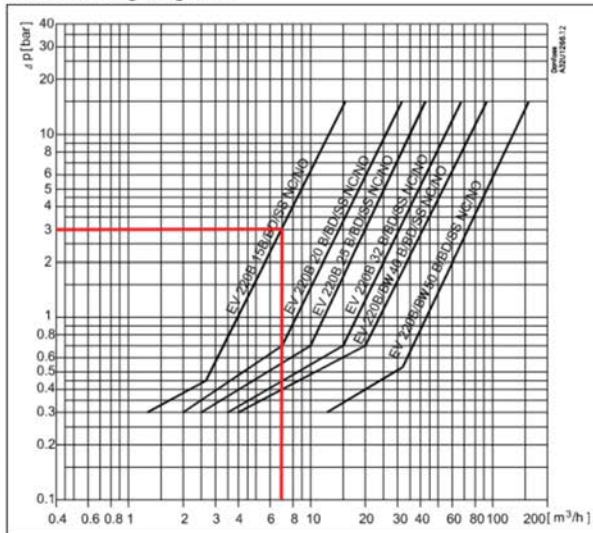
Bild 5: Leistungsdiagramm
