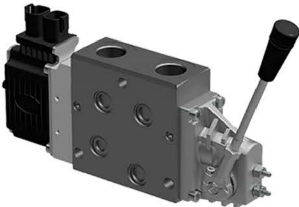
PVSKM slice
