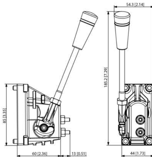
PVM dimensions
