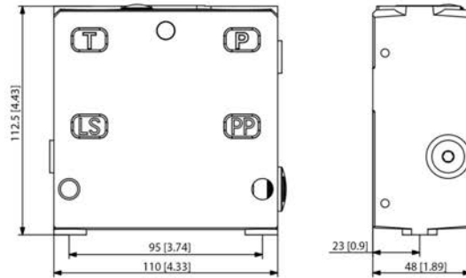
PVP inlet module dimensions
