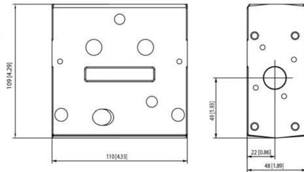
PVSKM module dimensions
