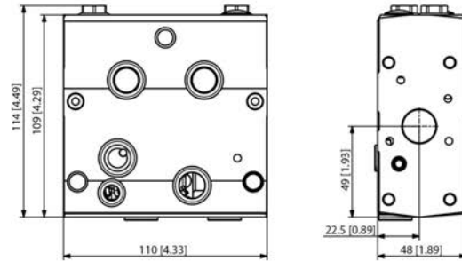
PVB 32 dimensions
