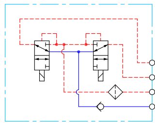
PVEO/PVEO-DI schematic
