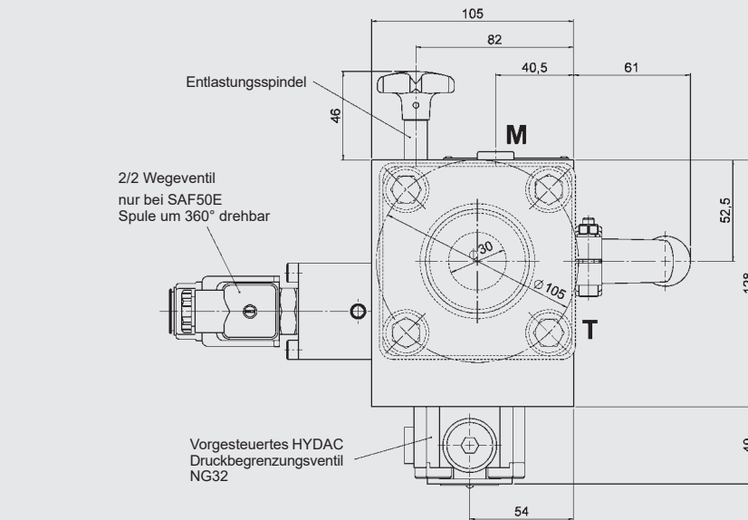
Vorgesteuertes HYDAC Druckbegrenzungsventil NG32
