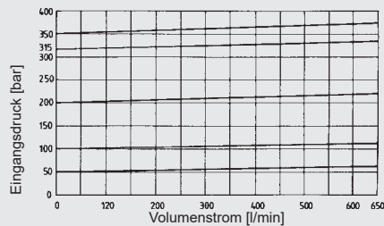
Vorgesteuertes HYDAC Druckbegrenzungsventil NG32
