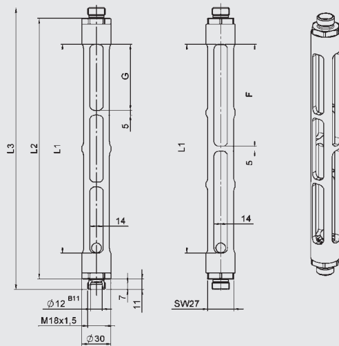
FSAR ohne Befestigungsmutter
