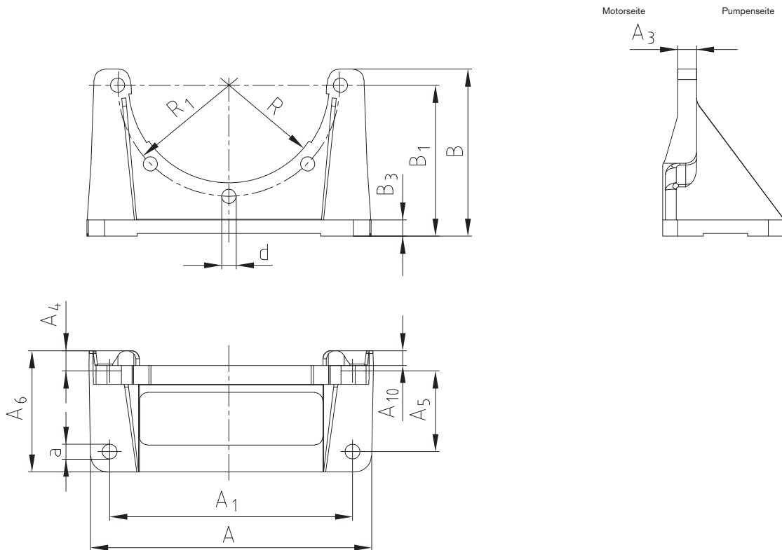
Fußflansch PTFL *
