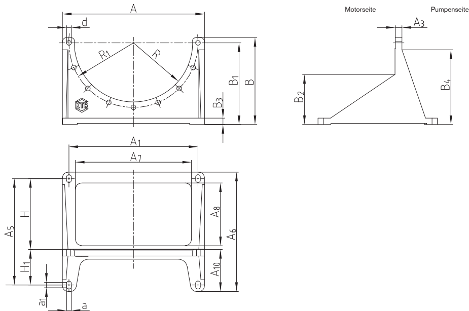
Fußflansch PTFS *
