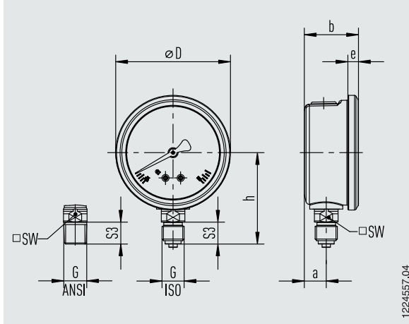
NG 50 [2"] und NG 63 [2 ½"], Anschluss radial unten
